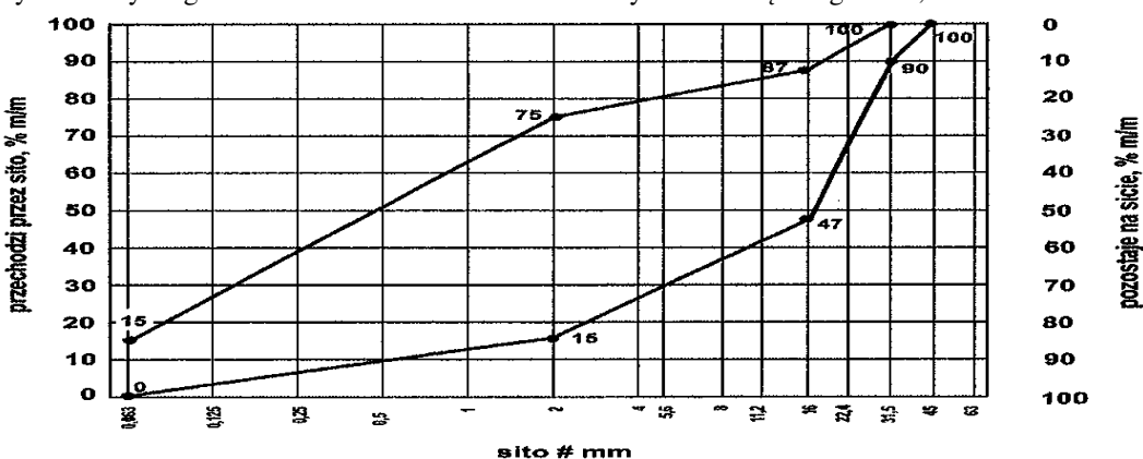
Rys. 3. Krzywe graniczne uziarnienia mieszanki kruszywa niezwiązanego 0/31,5 mm do nawierzchni
