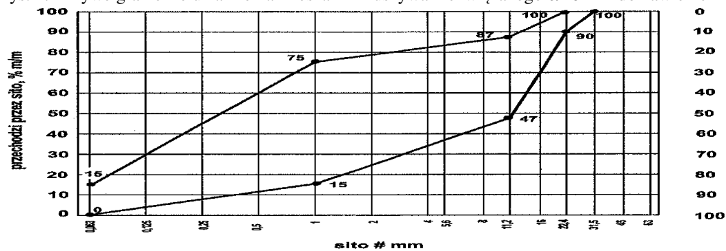
Rys. 2. Krzywe graniczne uziarnienia mieszanki kruszywa niezwiązanego 0/22,4 mm do nawierzchni
