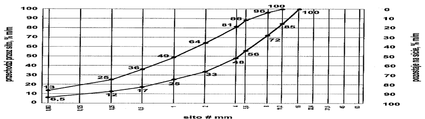
Rys. 4. Krzywe graniczne uziarnienia mieszanki mineralnej 0/11,2 mm
