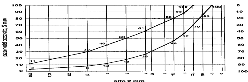
Rys. 1. Krzywe graniczne uziarnienia mieszanki mineralnej 0/31,5 mm
