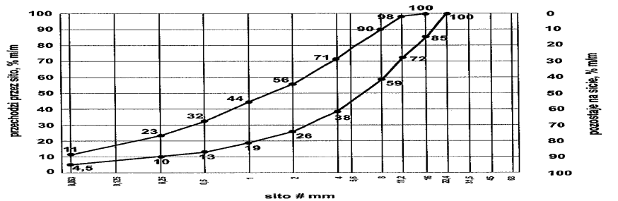
Rys. 3. Krzywe graniczne uziarnienia mieszanki mineralnej 0/16 mm
