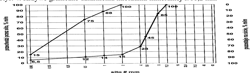
Rys. 5. Krzywe graniczne uziarnienia mieszanki mineralnej 0/8 mm
