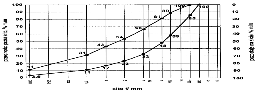
Rys. 2. Krzywe graniczne uziarnienia mieszanki mineralnej 0/22,4 mm
